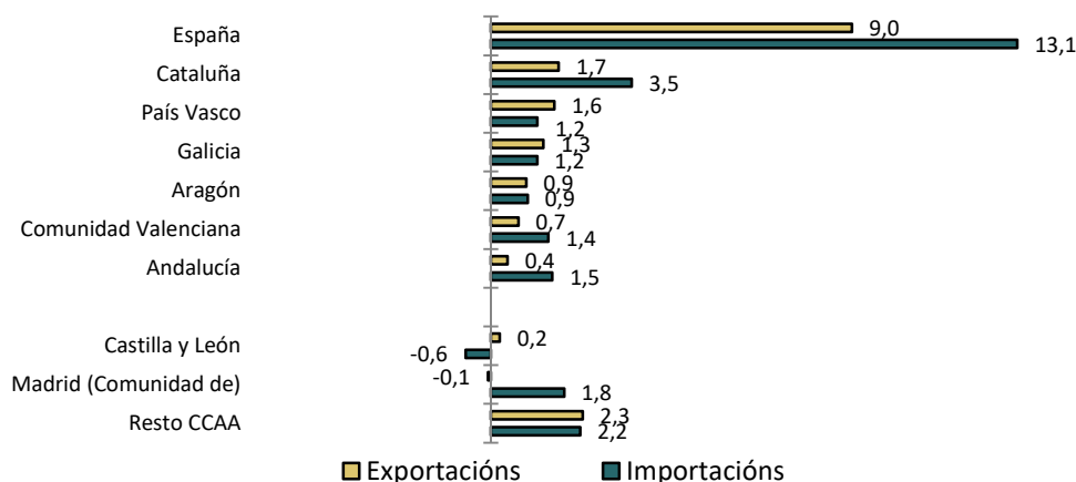
Gráfico 3. Comercio exterior por Comunidades Autónomas Outubro 2018. Principais achegas á taxa do total en %
