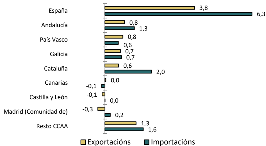
Gráfico 4. Comercio exterior por Comunidades Autónomas Xaneiro-outubro 2018. Principais achegas á taxa do total en %
